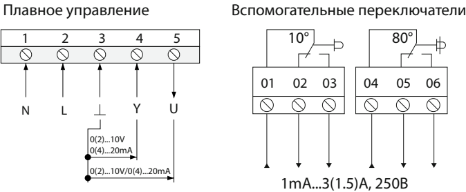
Настройка функций для DIP-переключателя S4
