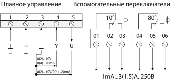
Настройка функций для DIP-переключателя S4
